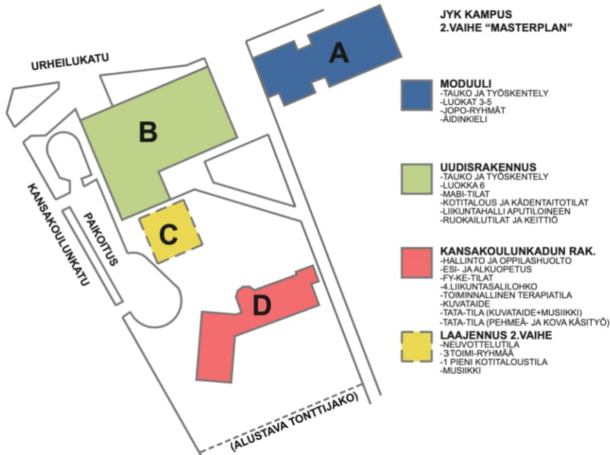
Kuva 1, JYK Vaiheen 2 valmistuttua koulutoiminnan käytössä olevat rakennukset.
